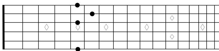
Dm9/A
