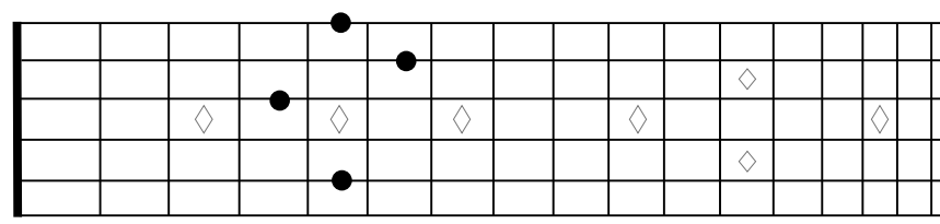
G13b9
