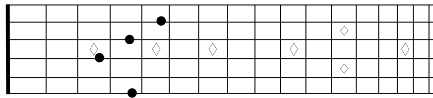
G7b5
