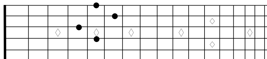
G9/D
