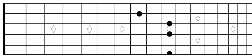
Dm11
