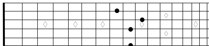
G7b5
