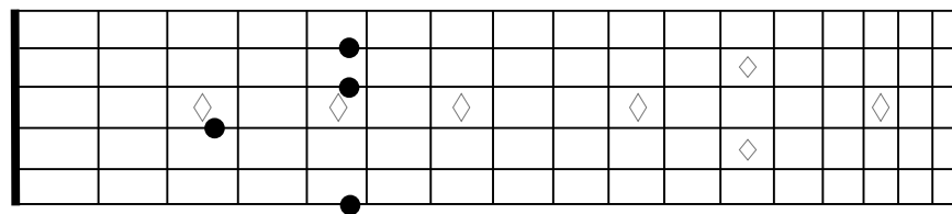
Dm11
